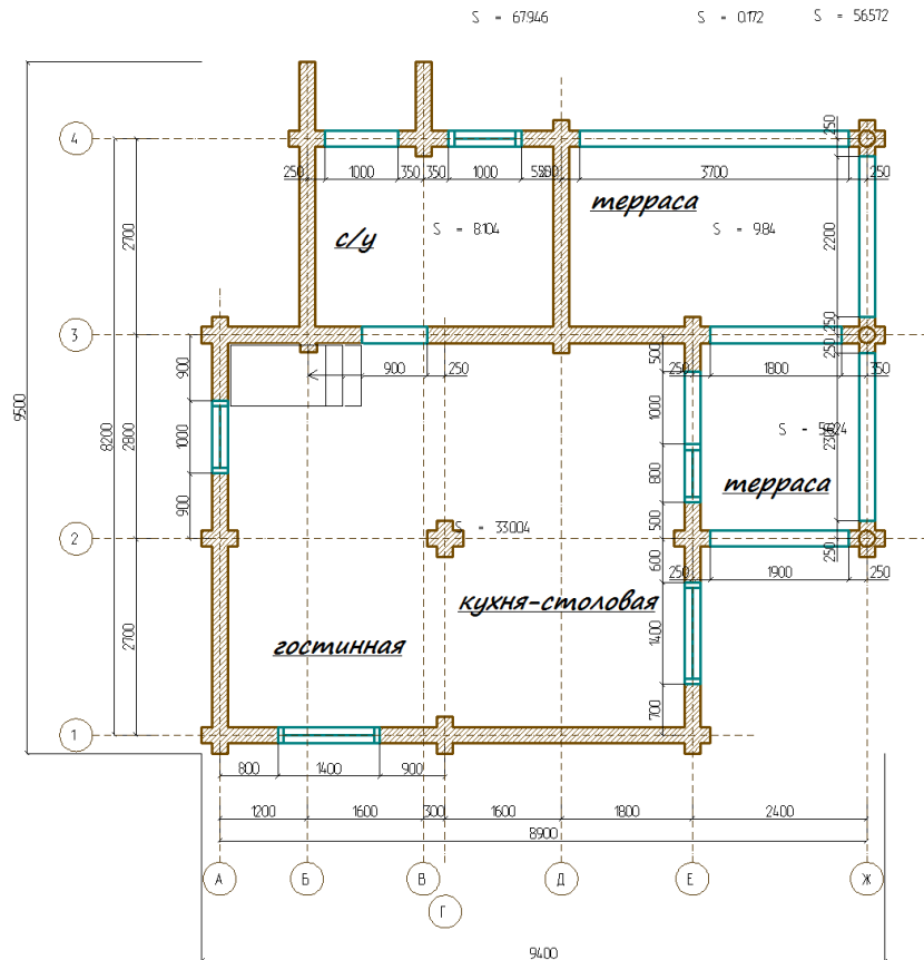
Планировка 1-го этажа
