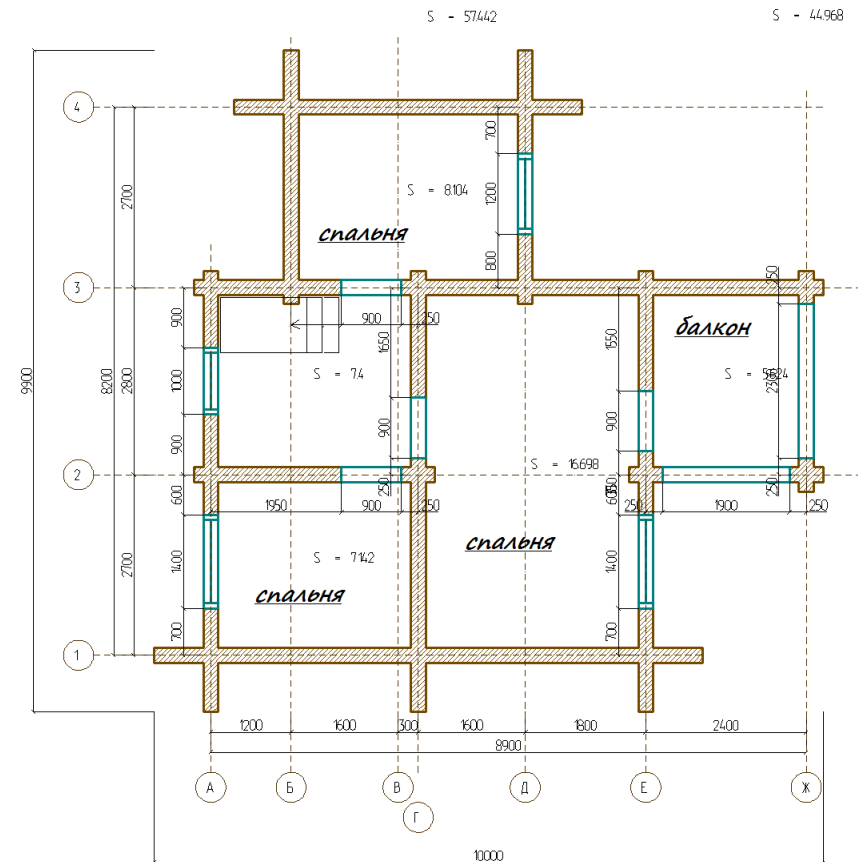
Планировка 2-го этажа
