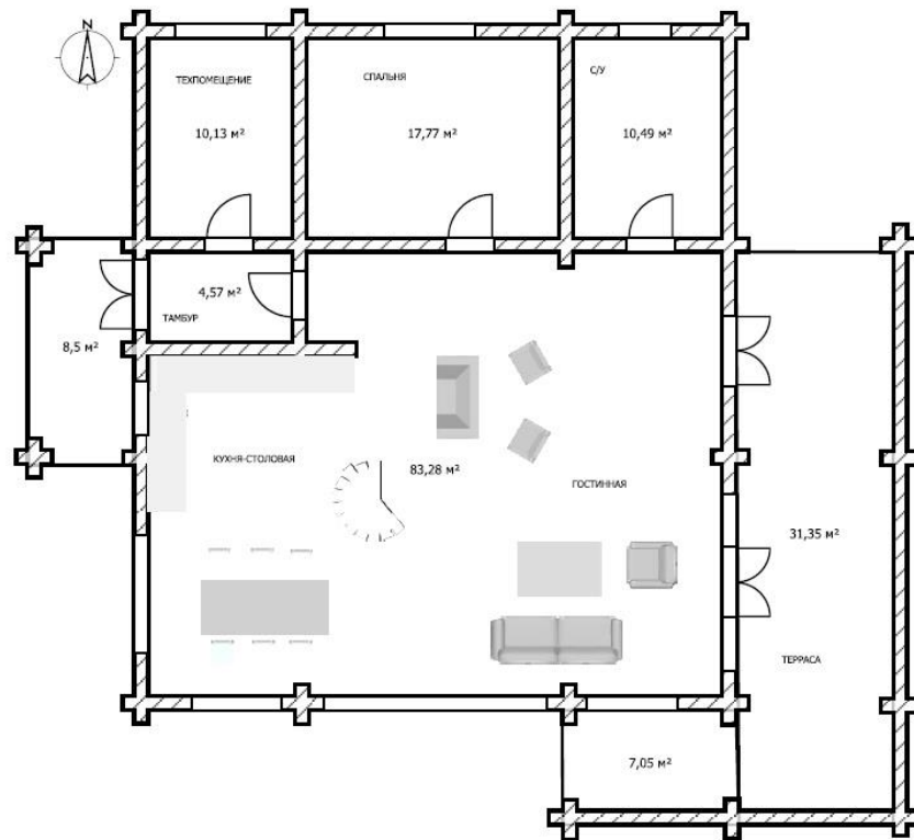
Планировка 1-го этажа
