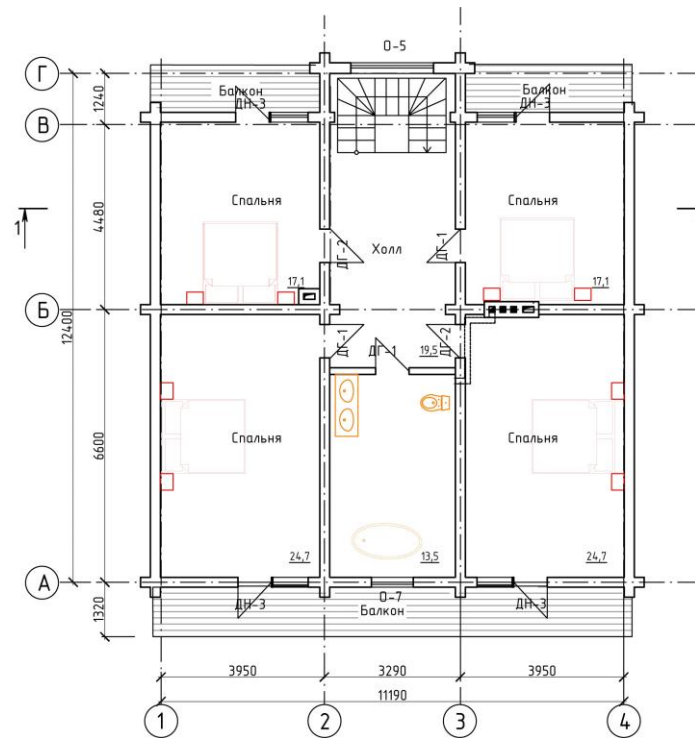
Планировка 2-го этажа
