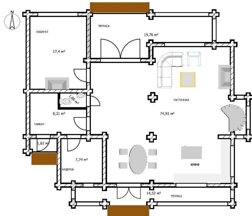
Планировка 1-го этажа
