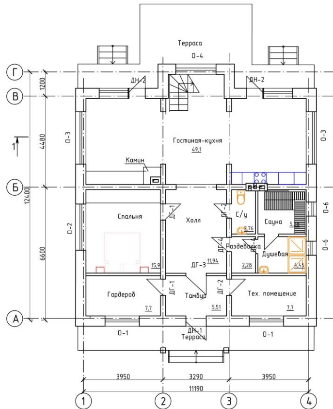
Планировка 1-го этажа
